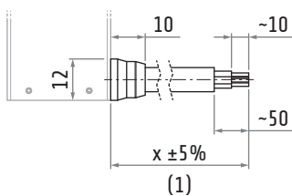
FCT2L03...D
